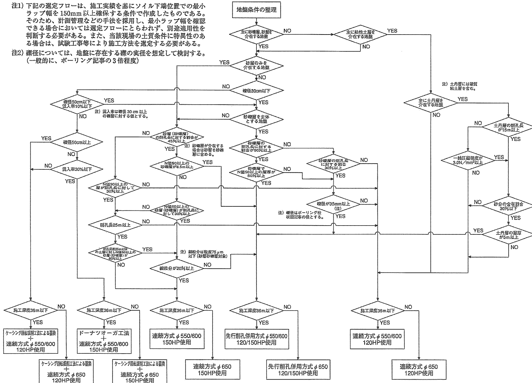
550 S MW造壁順序及びアースオーガ選定フロー
